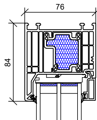
Schnitt C
