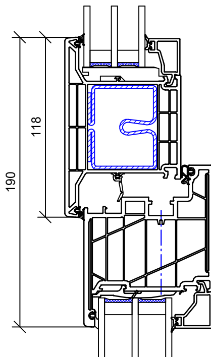
Schnitt A
