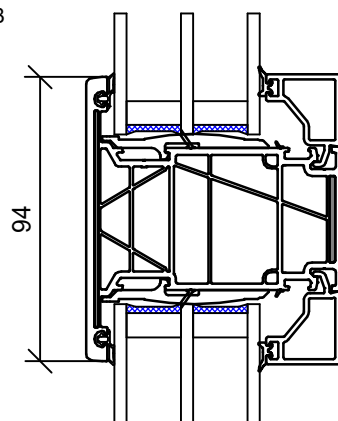
Schnitt B
