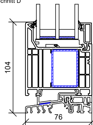
Schnitt D
