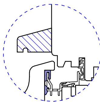
Wetterschenkel (WF)
