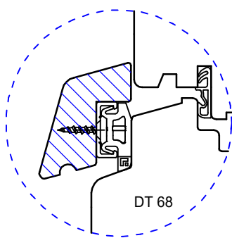
Regenschiene mit Holzabdeckung (RH)
