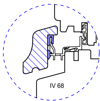
Regenschiene mit Holzabdeckung (RH)
