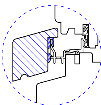
mit Wetterschenkel (RW)
